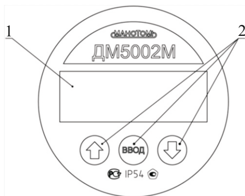
Рисунок 2.1 – Панель индикации ДМ5002М
