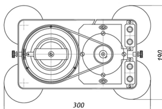
Электропривод ИПС для МГП-0,2...0,5
