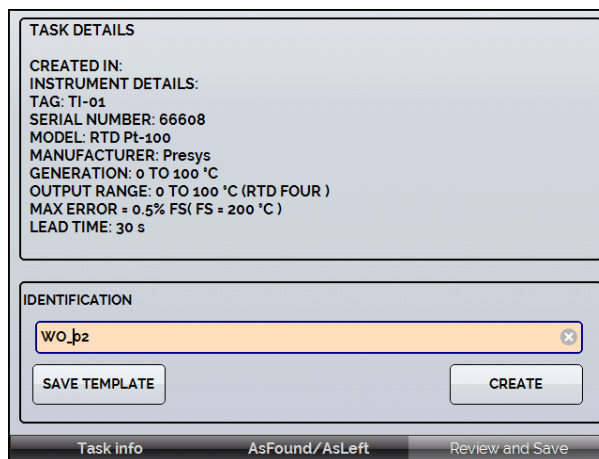
Рис. 27 – Создание задания
